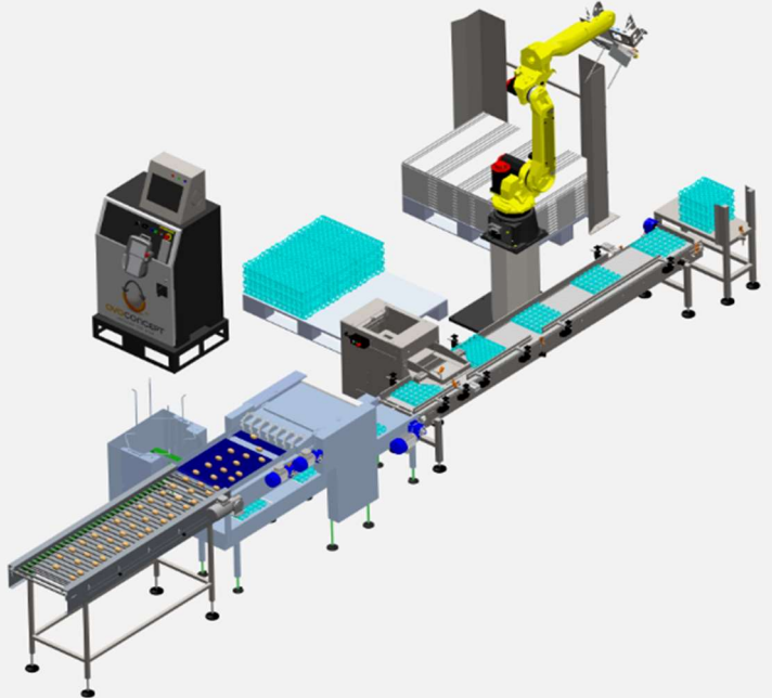
ROBOT JUNIOR SE23
